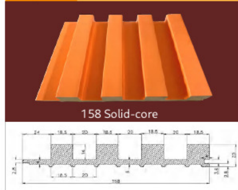
型号/Model HL158
