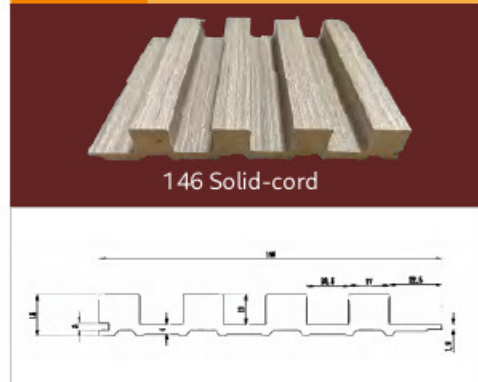
型号/Model HL146
