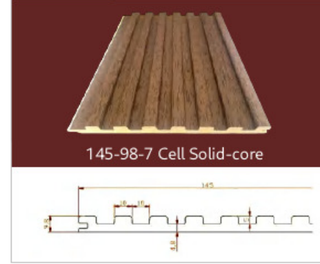
型号/Model HL145-98-7
