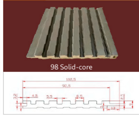
型号/Model HL98
